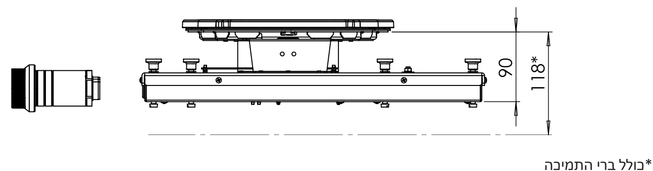
מבט צדדי
