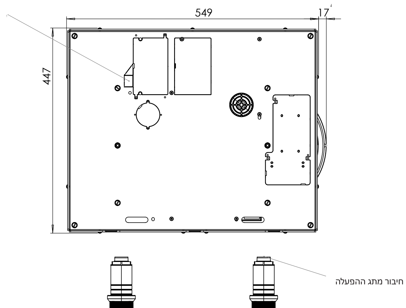
מבט תחתון
