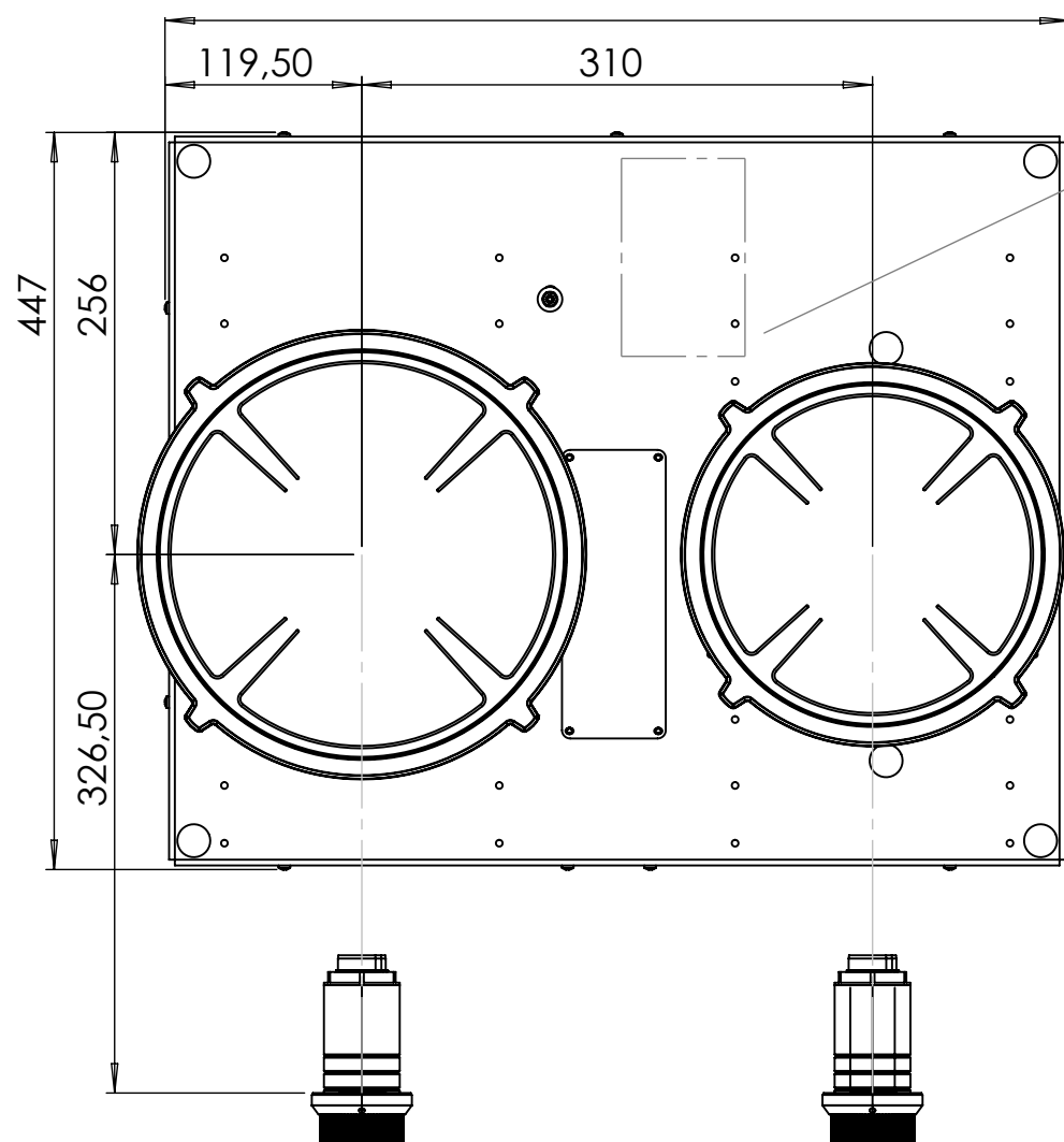
מבט עליון
