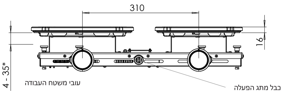
מבט חזיתי
